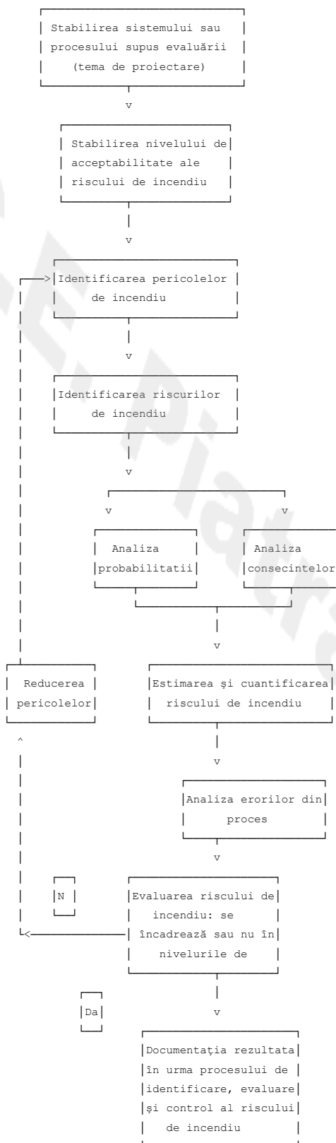
Schema logica de management al riscurilor de incendiu în faza de proiectare
