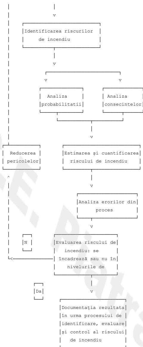
Schema logica de management al riscurilor de incendiu în faza de proiectare
