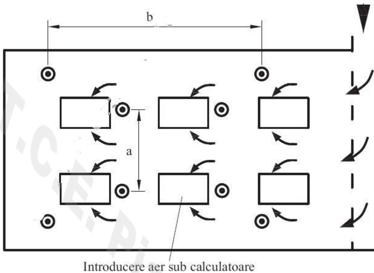
Figura 3.17 Amplasarea detectoarelor într-o încăpere cu circulația internă a aerului
