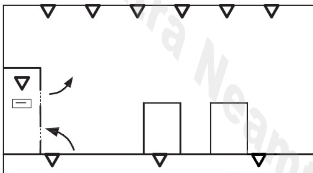
Figura 3.18 Amplasarea detectoarelor într-o încăpăre cu utilaje răcite cu aer
