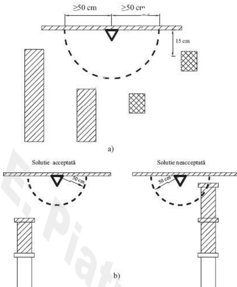
Figura 3.4 Amplasarea detectorului față de elemente de construcții
