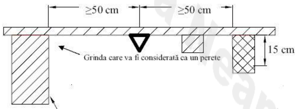
Figura 3.4 Amplasarea detectorului față de elemente de construcții
