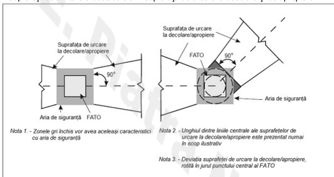
Figura 1.9 - Lățimea suprafeței de urcare la decolare/apropiere
