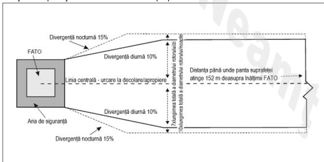
Figura 1.10 - Suprafața de tranziție pentru FATO cu procedură de apropiere PinS cu VSS
