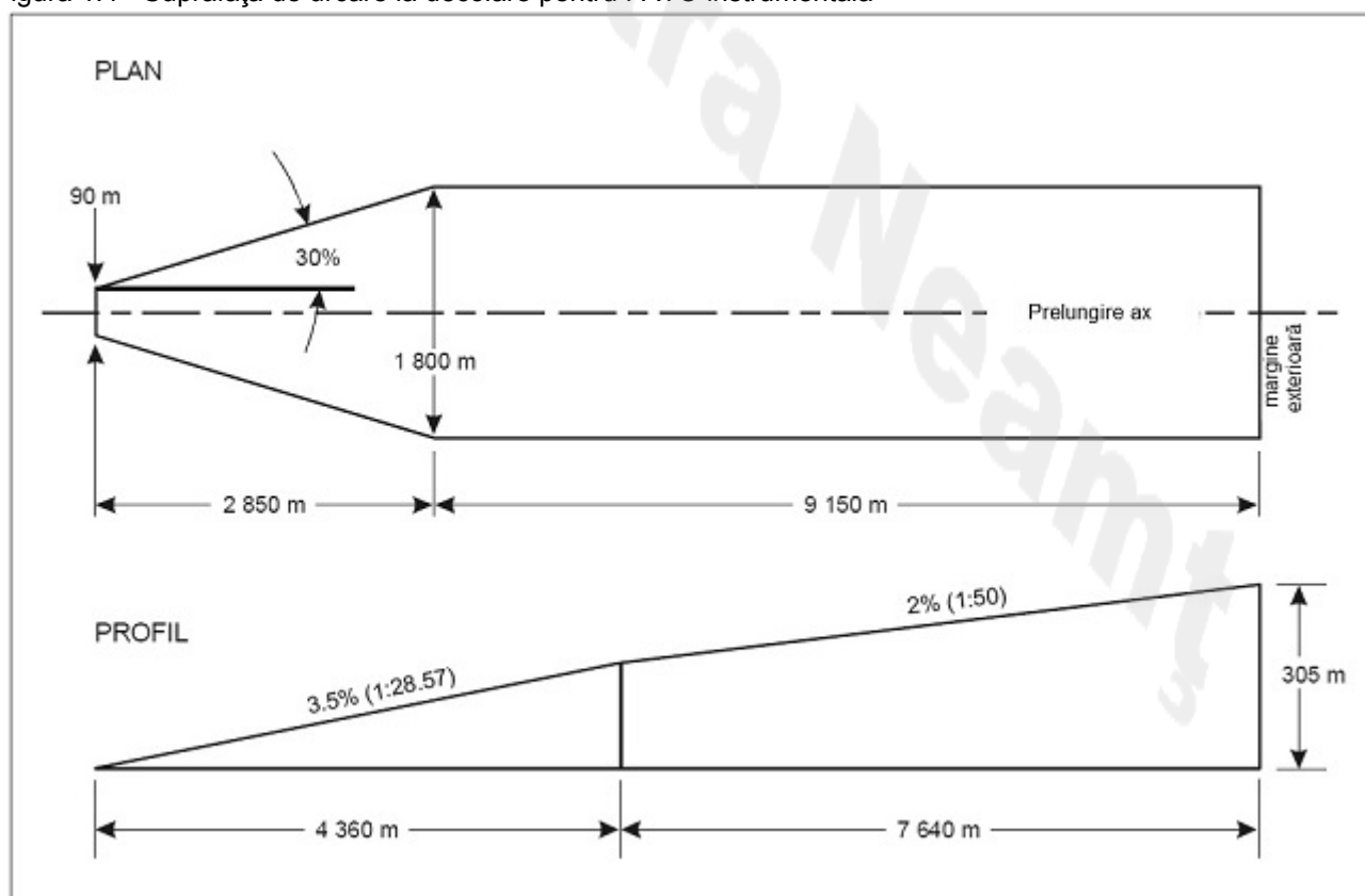
Figura 1.5 - Suprafața de apropiere pentru FATO cu apropiere de precizie
