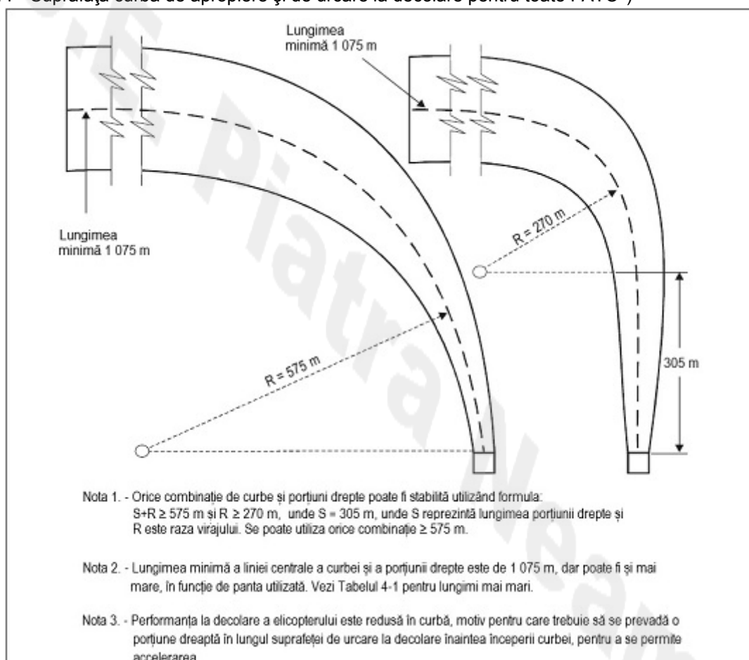
Figura 1.11 - Suprafața curbă de apropiere și de urcare la decolare pentru toate FATO*)
