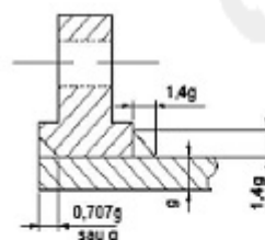
4. FLANȘĂ PLATĂ PT. SUDAT
