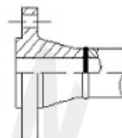
2. FLANȘĂ CU GĂT PT. SUDARE
