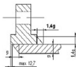
3. FLANȘĂ PLATĂ PT. SUDAT
