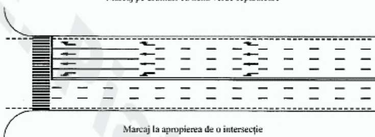
Marcaj pe drumuri cu zonă verde separatoare
