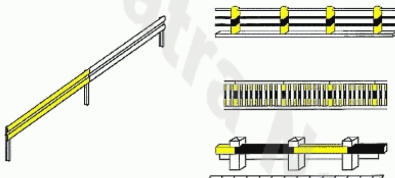
Marcaje pe parapete
