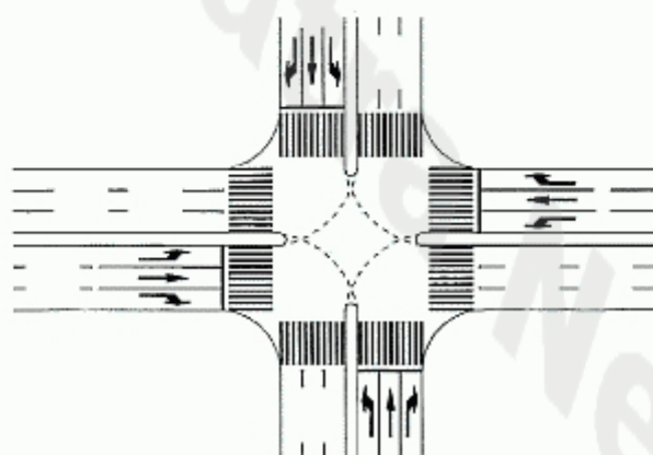
Marcaj de ghidare în intersecție
