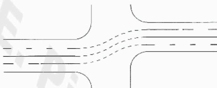
Marcaj de ghidare la traversarea unei intersecții
